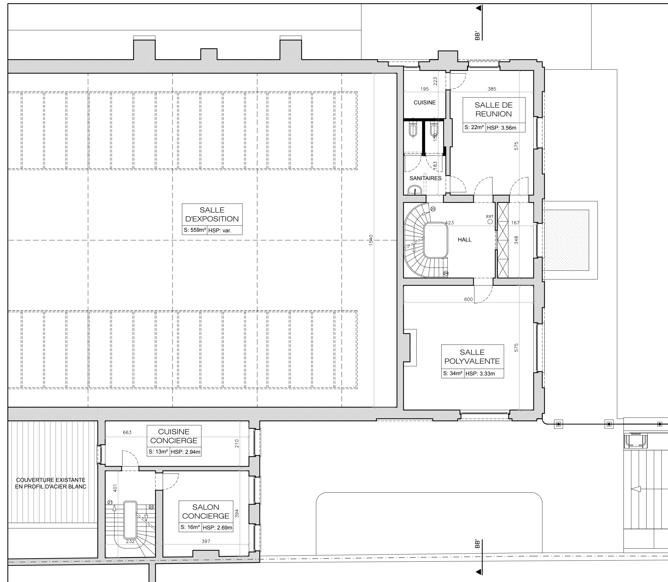
PLAN 1er ETAGE (1/100)
