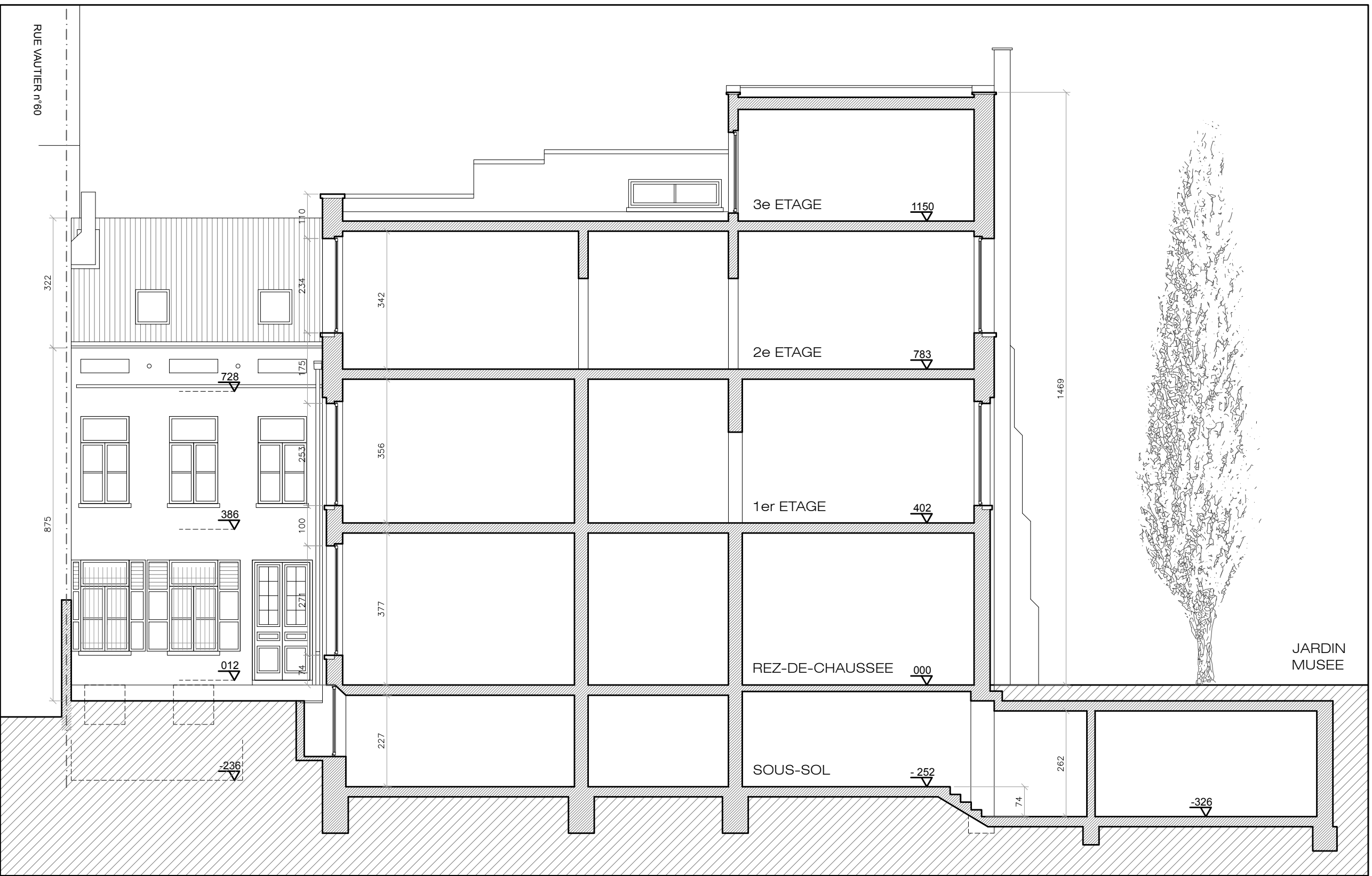
COUPE BB' (1/100)
