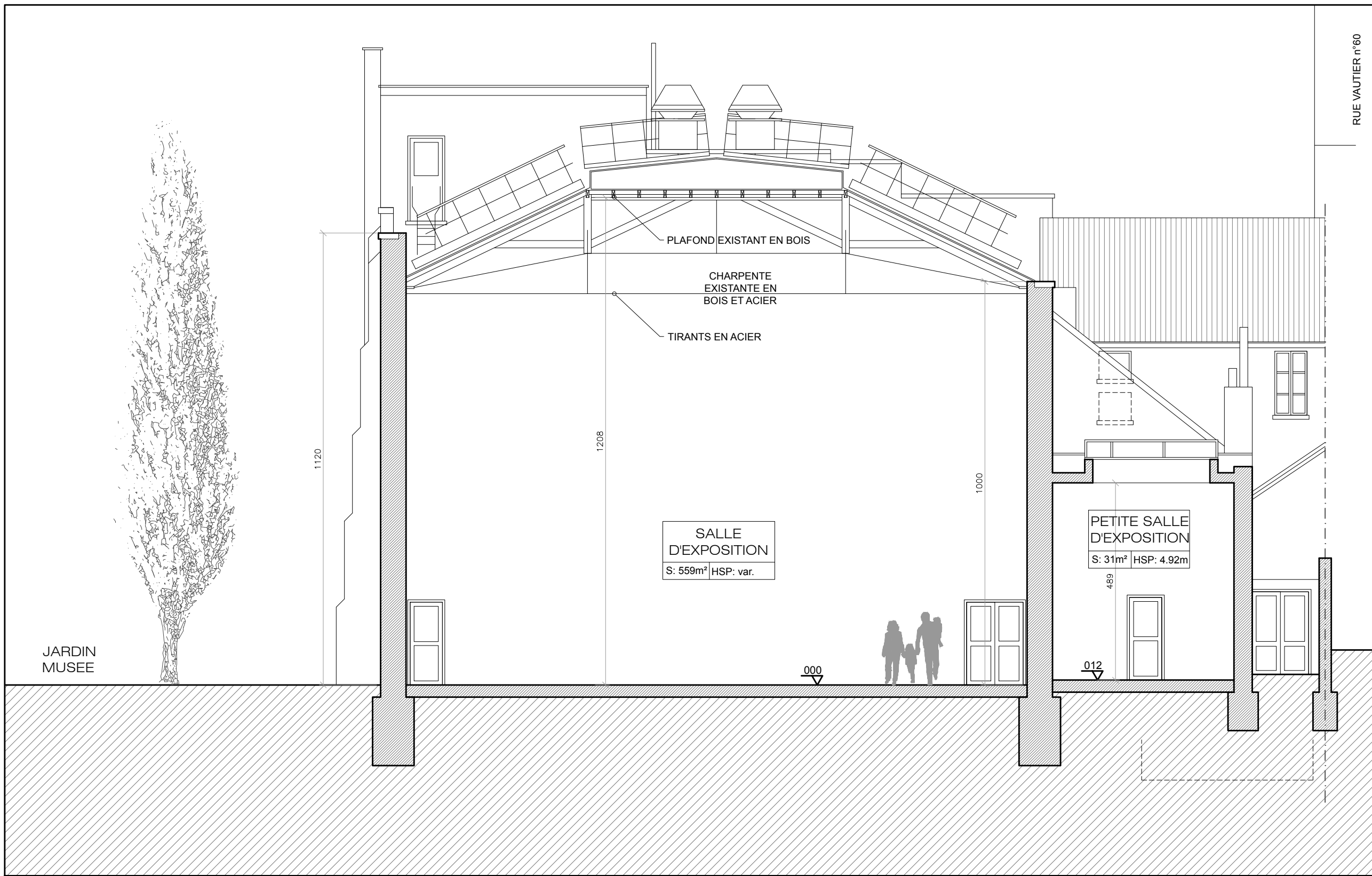
COUPE AA' (1/100)
