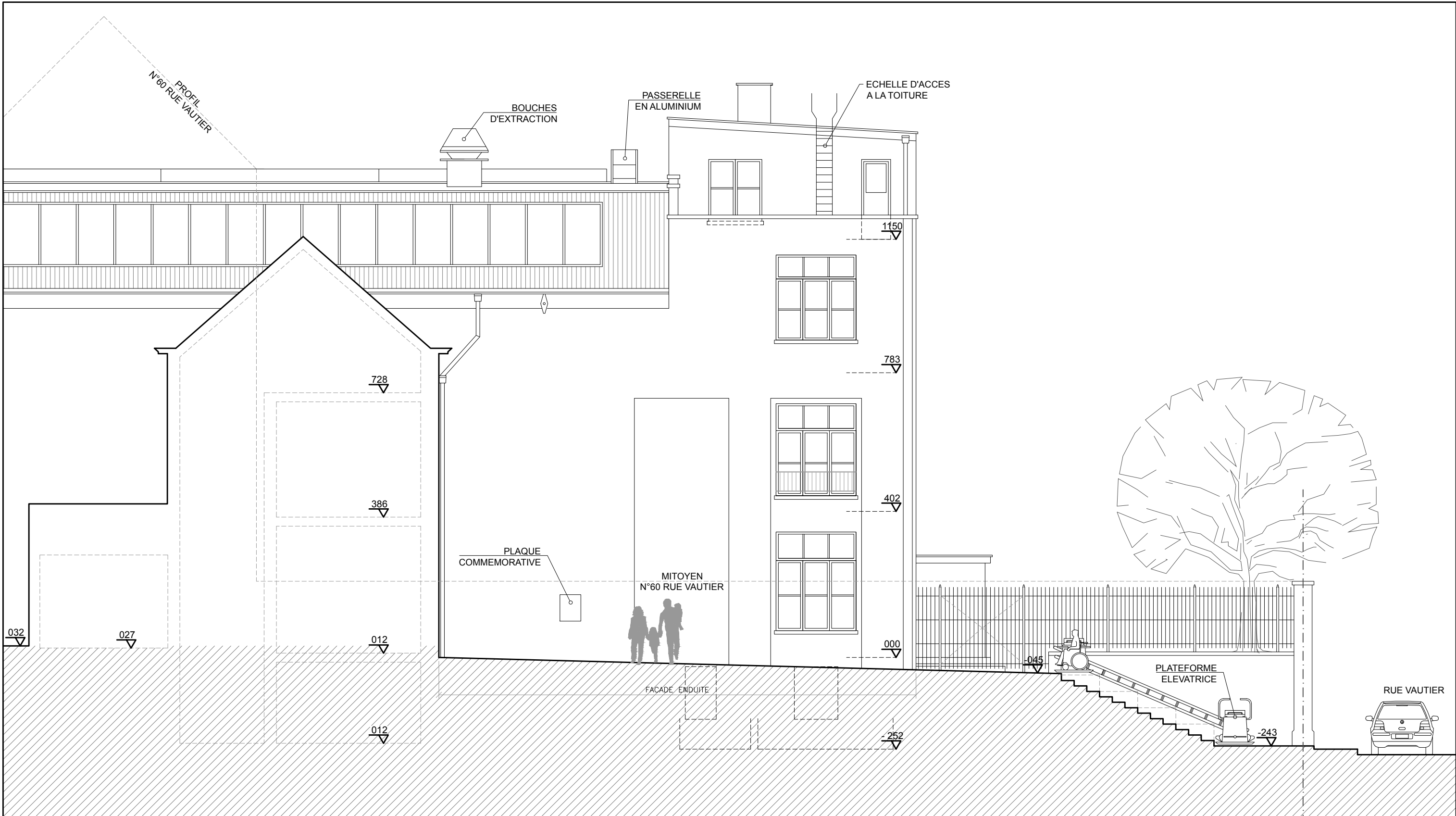
FACADE LATÉRALE GAUCHE (1/100)
