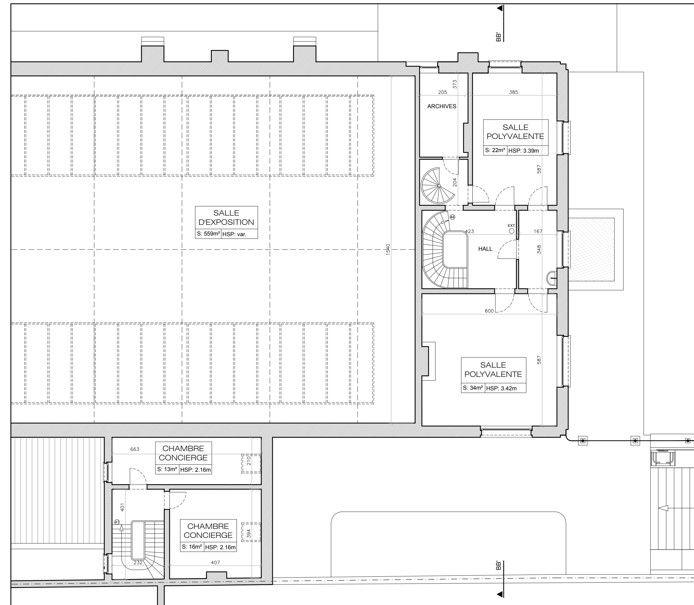
PLAN 2e ETAGE (1/100)
