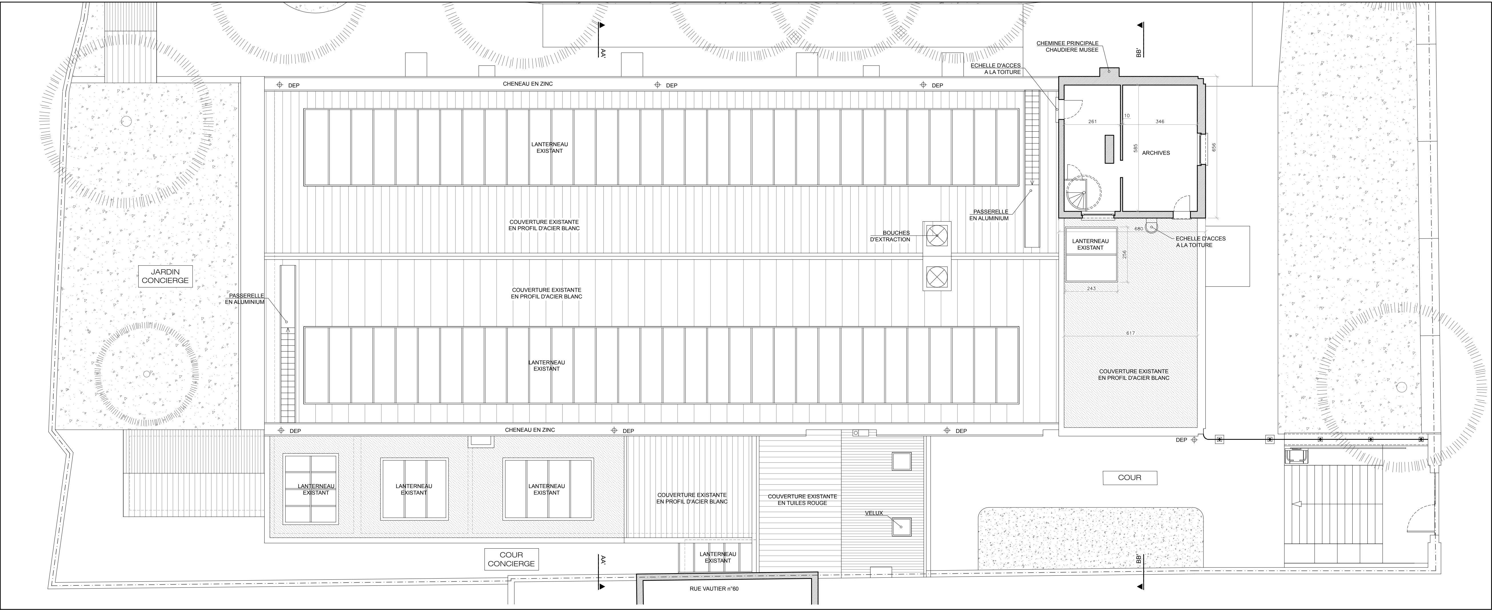
PLAN TOITURES (1/100)
