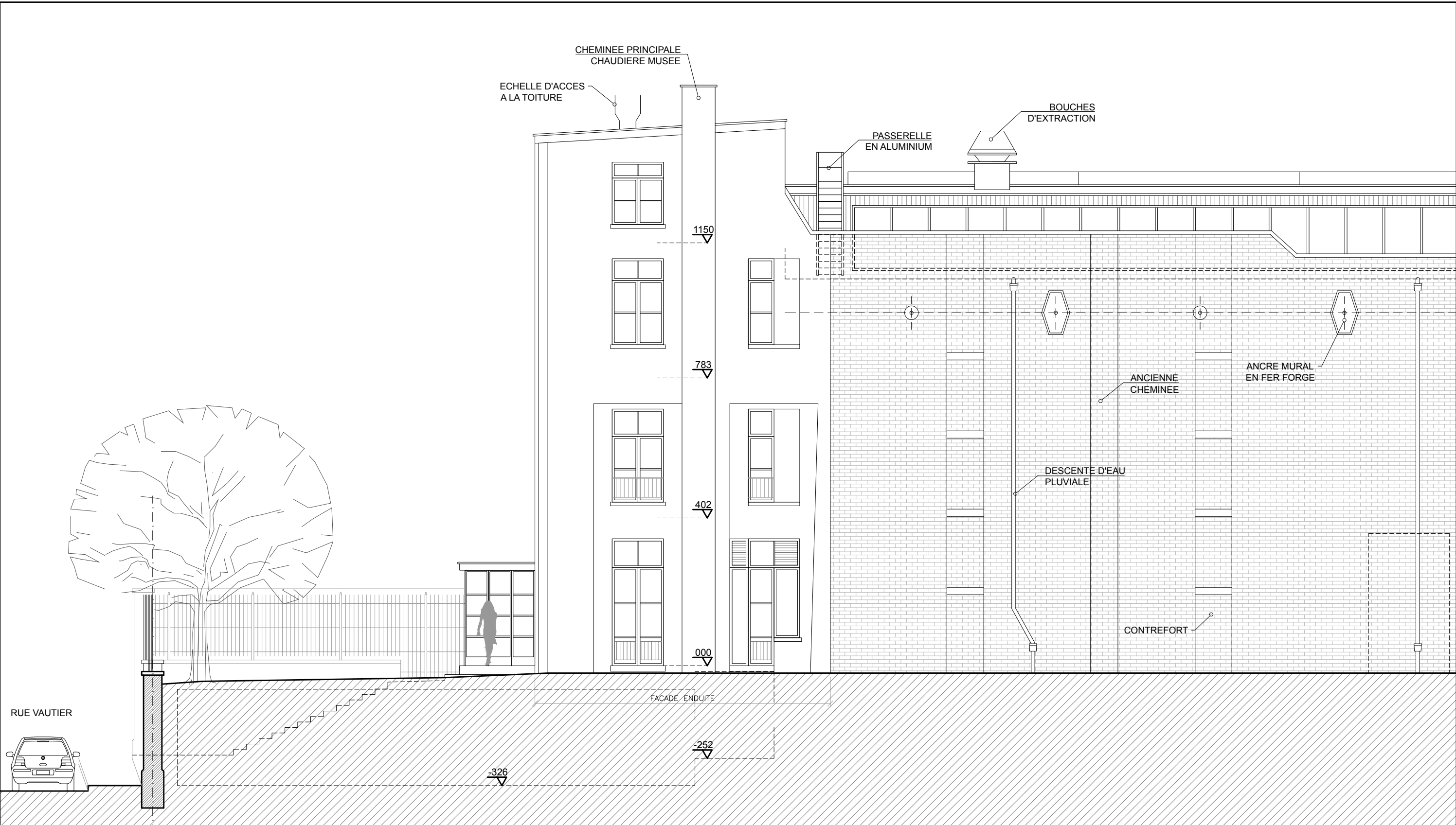
FACADE LATÉRALE DROITE (1/100)
