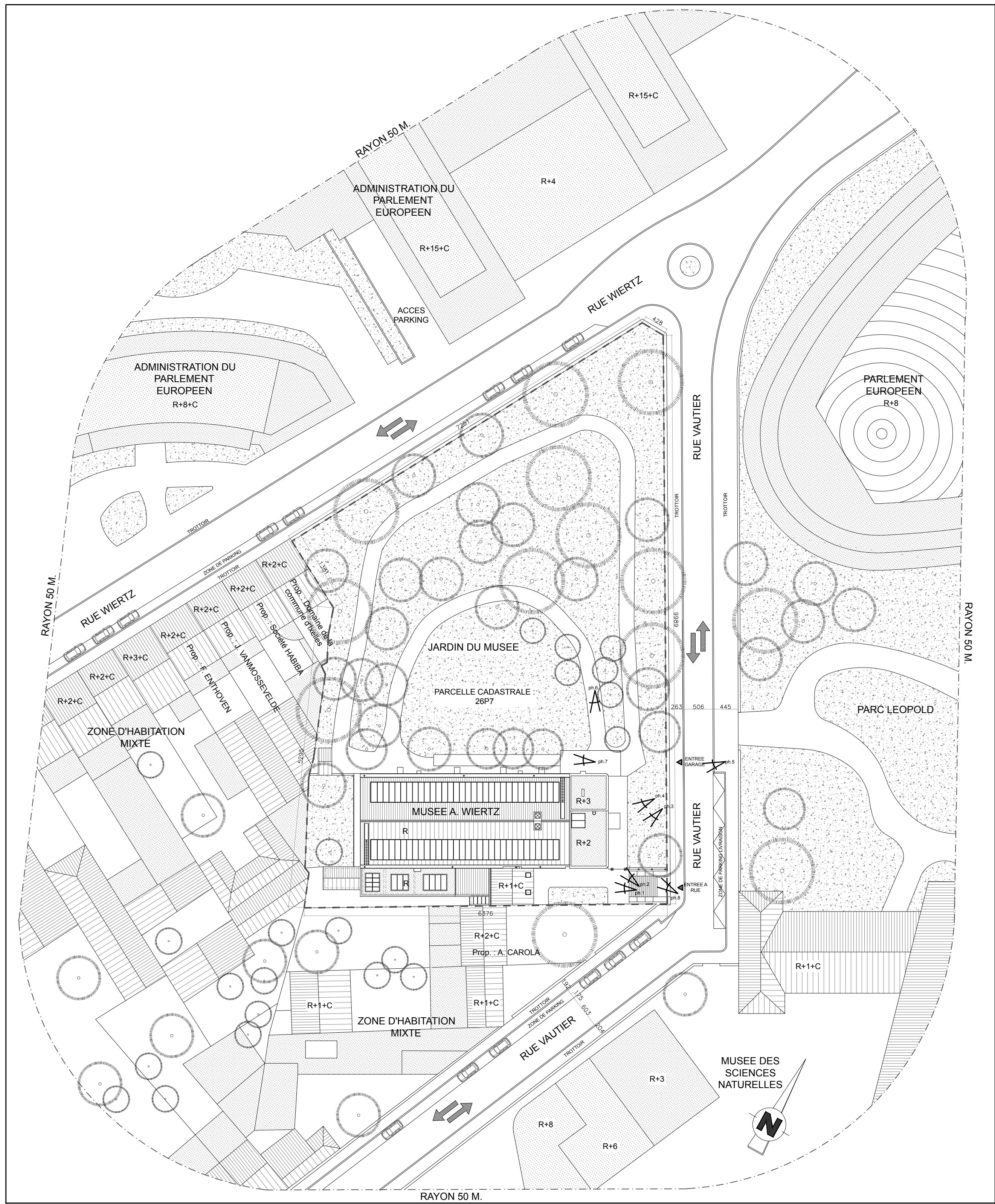
PLAN D'IMPLANTATION (1/500)
